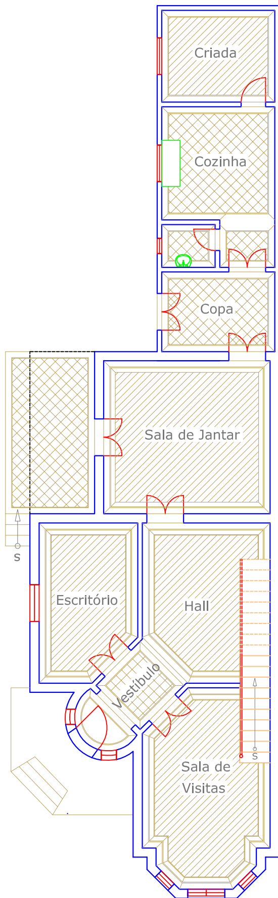
TERREO
