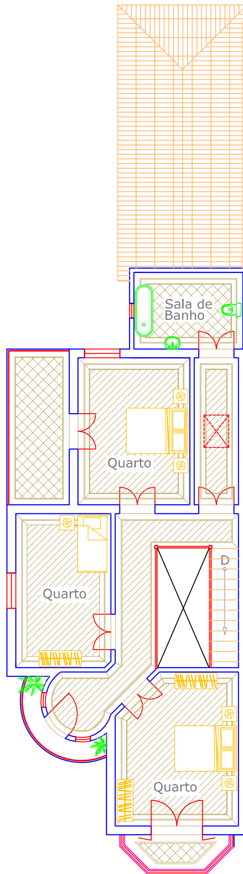
SUPERIOR
